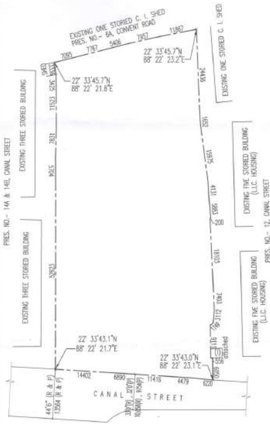
SITE PLAN SCALE-1:800
